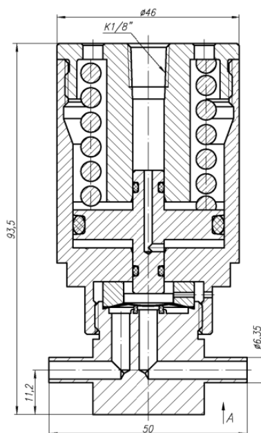
Габаритные, установочные и присоединительные размеры
